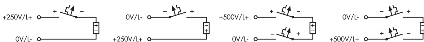
Tilslutningseksempel for 250V=, enkelt pol
