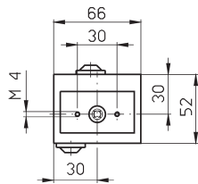
Schalterstirnseite Front view
