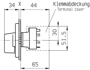
Schaltereinsatz Insert
